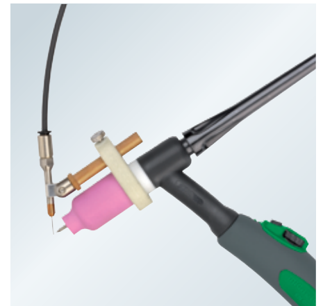
Kaltdrahtführung am Schweißbrenner montiert
