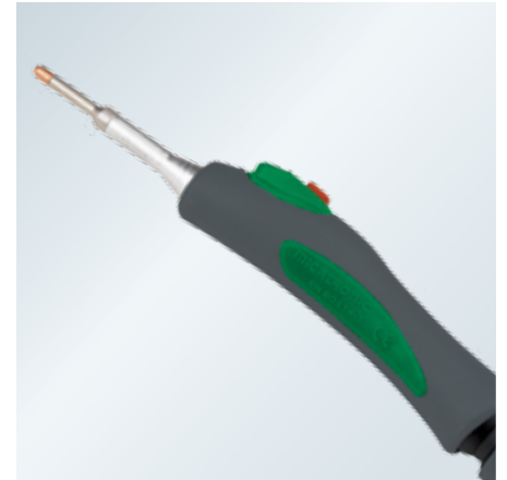
Kaltdraht-Pistole Ausgerüstet mit Start/Stop und Regelung der Drahtgeschwindigkeit am Griff
